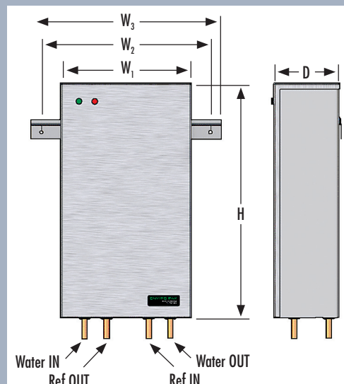
Enviro-Pak Dimensions
